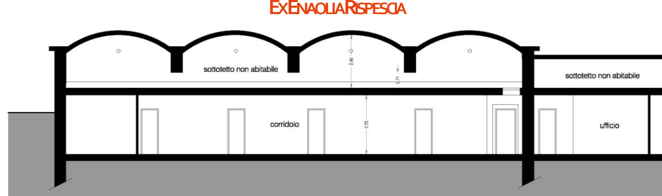
SEZIONE AA
